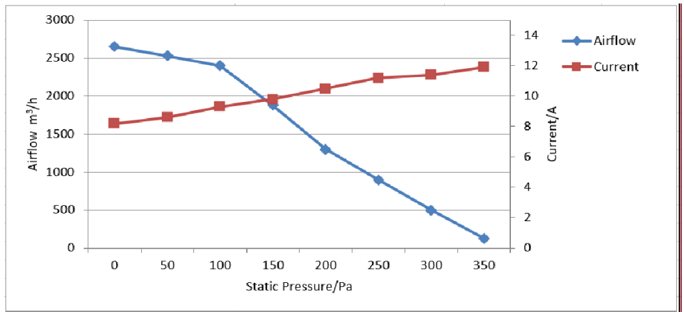
305mm 有刷轴流风机 24V DC 305mm Brush Axial Fan
