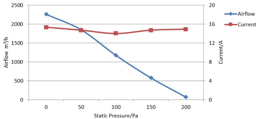
305mm 有刷轴流风机 12V DC 305mm Brush Axial Fan
