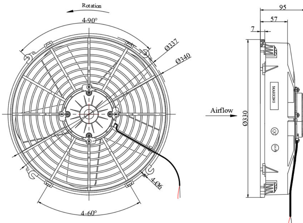
安装尺寸图 (单位: 毫米) Dimension (Unit: mm)
